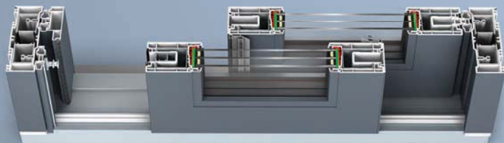
Schema A - Horizontalschnitt
